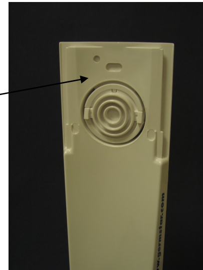
Détail de la glissière de fixation
